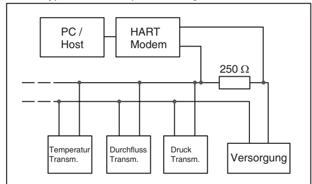
Bild 3: Typische Multidrop-Anordnung
