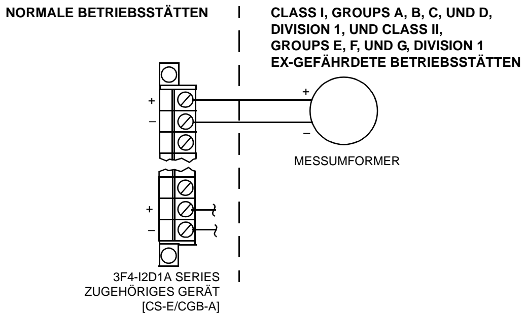
Abbildung 7. FIO-Subsystem - Schleifendiagramm
